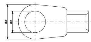
Cable lug DIN 46235: 1980-07
